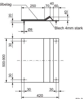
Standvorrichtung für Weiten- und Schnellwettbewerb
